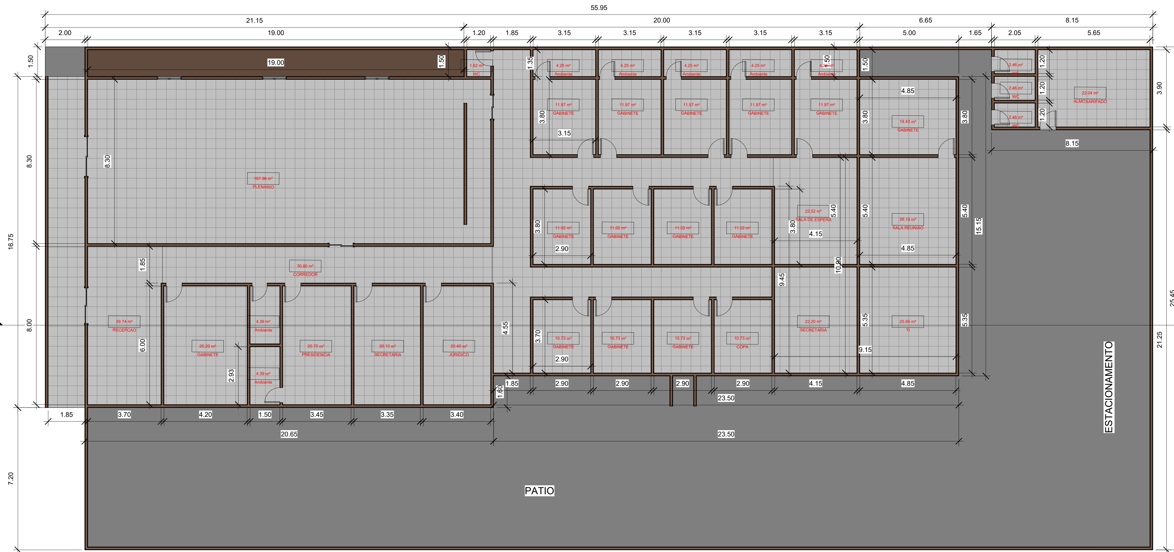
1 Planta Baixa 1 : 100
